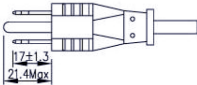
NEMA5-15P (15A)
